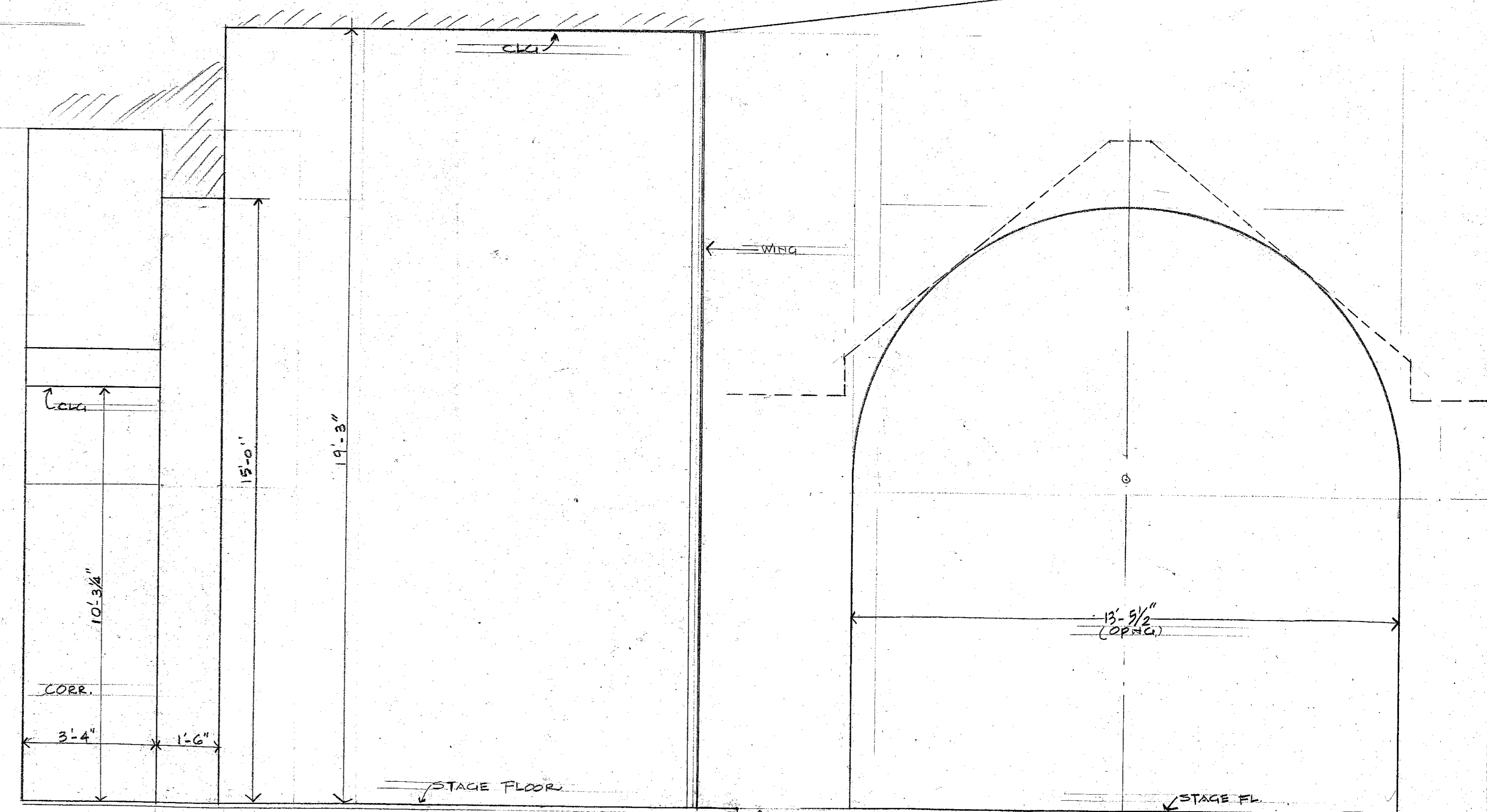
SECTION A-A
